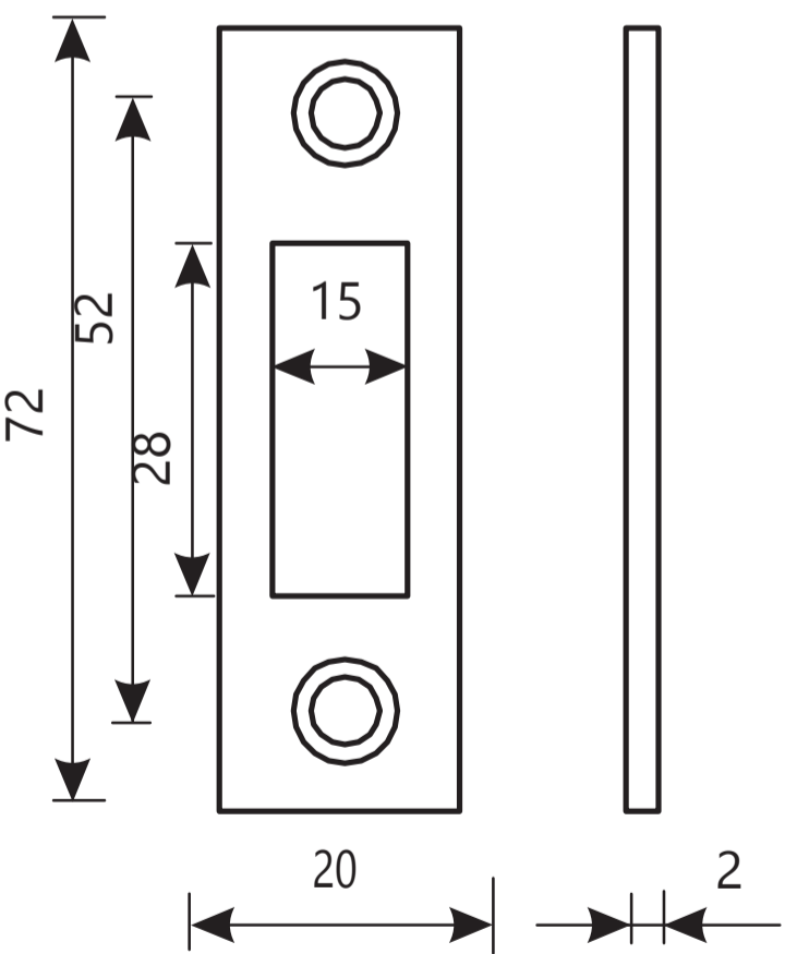
Ответная планка
